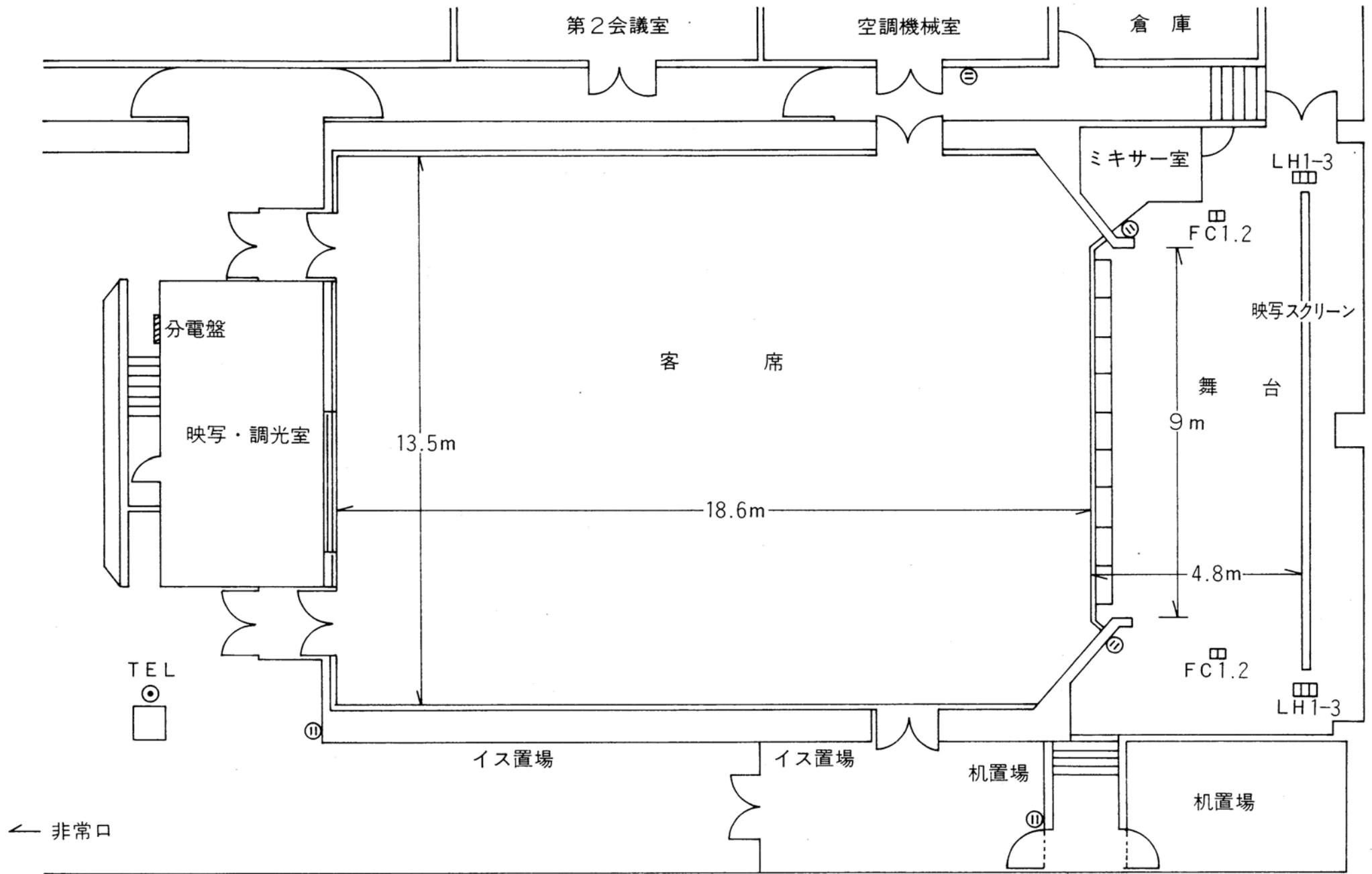
■ 講堂平面図 縮尺 1/100
